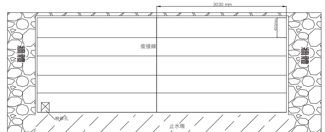
覆壁立面展開示意图 (對縫施工)
