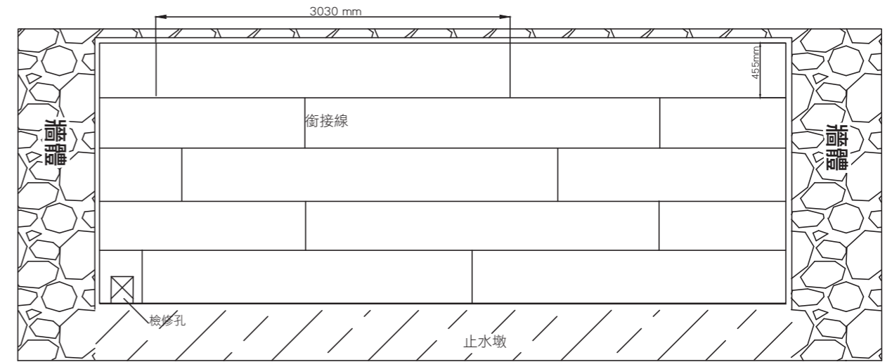
覆壁立面展開示意图 (搭接施工)
